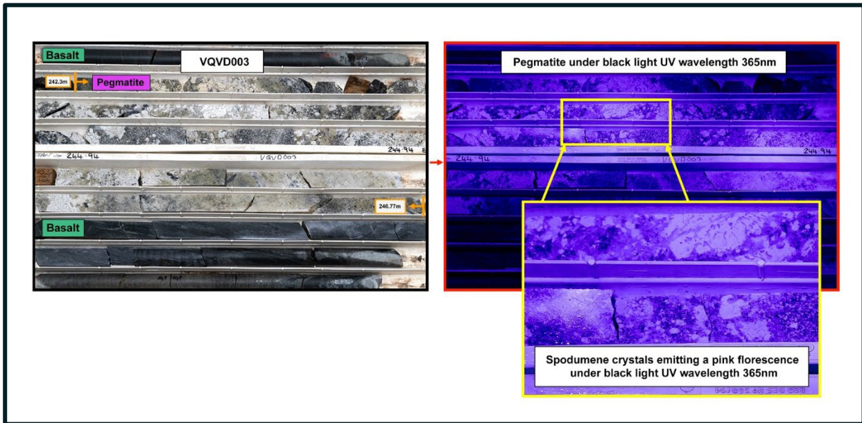
Abbildung 1 – Diamantkern von VQVD003 mit Kennzeichnung von Pegmatit, der von 242,3 – 246,77 m unter UV-Wellenlänge 365nm (Schwarzlicht) durchgeschnitten wurde. Spodumen fluoresziert unter UV-Licht von 242,3 – 245,5 m orange-pink.
