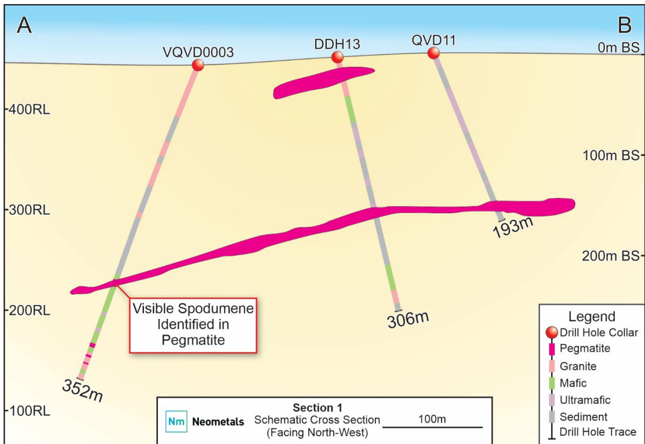
Abbildung 4 – Querschnitt von historischen Diamantbohrlöchern auf Spargos mit protokollierten Pegmatiten.
