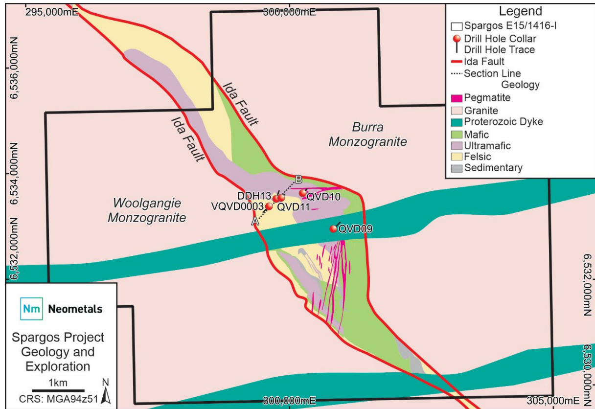
Abbildung 3 – Geologie von Spargos mit Geländekartierung und Lithiumexploration. Lage von Sektion 1 auf der Karte angezeigt.
