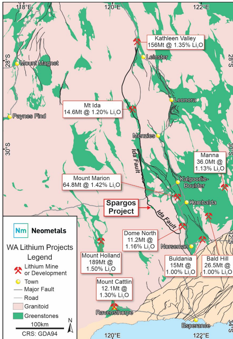
Abbildung 2 – Lage des Projekts Spargos im Verhältnis zu großen westaustralischen Lithiumminen oder -erschließungen in der Goldfields-Region (öffentlich zugängliche Lithiumressourcendaten vom Department of Mines, Industry Regulation and Safety, 1. Mai 2023).
